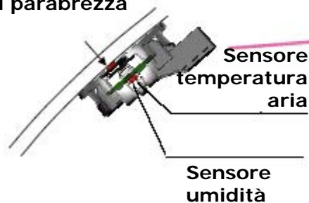
Sensore temperatura sul parabrezza
